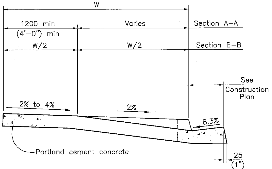
SECTION A-A & B-B
